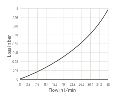
ПОТЕРИ НА ТРЕНИЕ ПОДВИЖНЫХ СОЕДИНЕНИЙ
