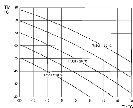
График 2 TM = температура воды на подаче в контур отопления Te = температура наружного воздуха Sth = кривая Kt
